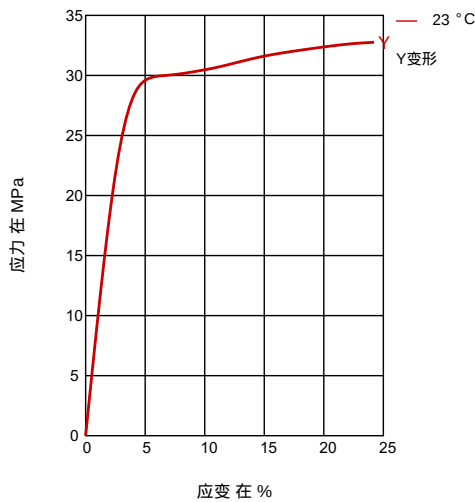
应力 - 应变.
